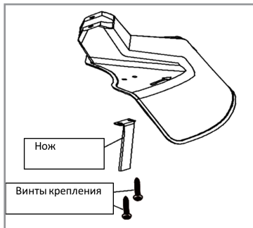
Рис. 2 Установка ножа для обрезки корда
