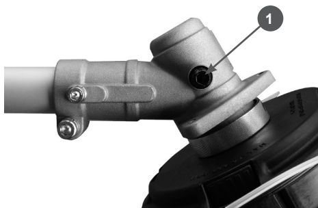
Рис. 17 Болт отверстия для смазки редуктора
