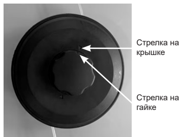
Рис.13 Совмещение стрелок
