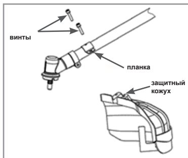
Рис. 3 Установка защитного кожуха
